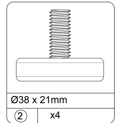
Adjustable glide Ajustable se deslizando TWTI0025
