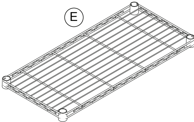
Mesh shelf(4) Tablette en treillis(4) T9491096STC050
