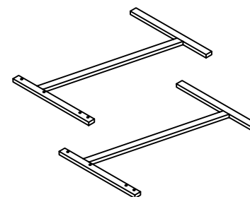
R SIDE FRAME Marco lateral CÔTÉ CADRE T9302096180
